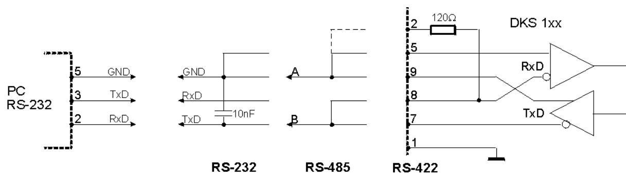
Rys. 3 Interfejs kanału szeregowego koncentratora
