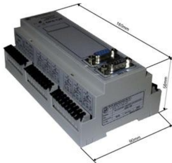
Rys. 2 Rysunek gabarytowy
